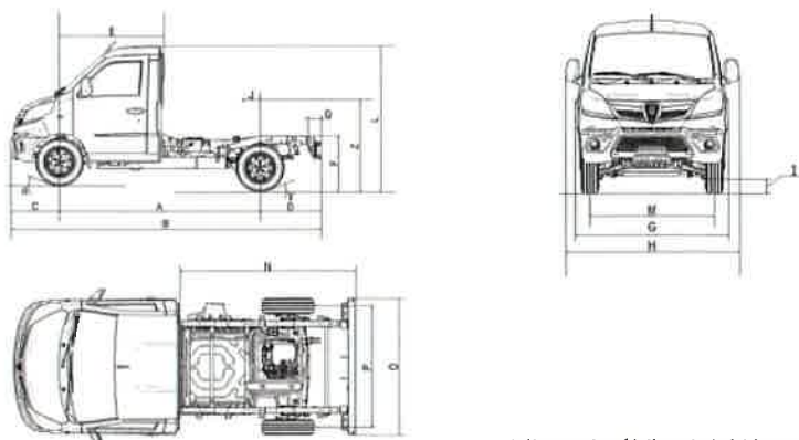
Nákresy odpovídají verzi s krátkým rozvorem.
